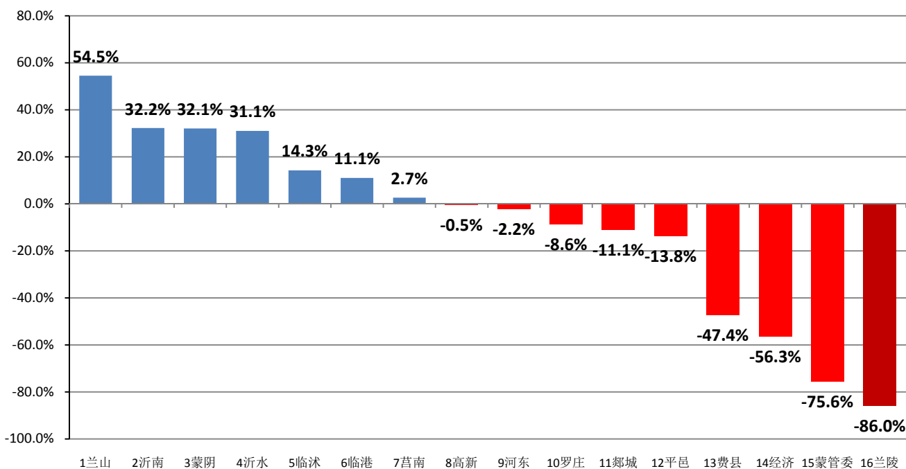
图 6 各县区总磷同比改善幅度
