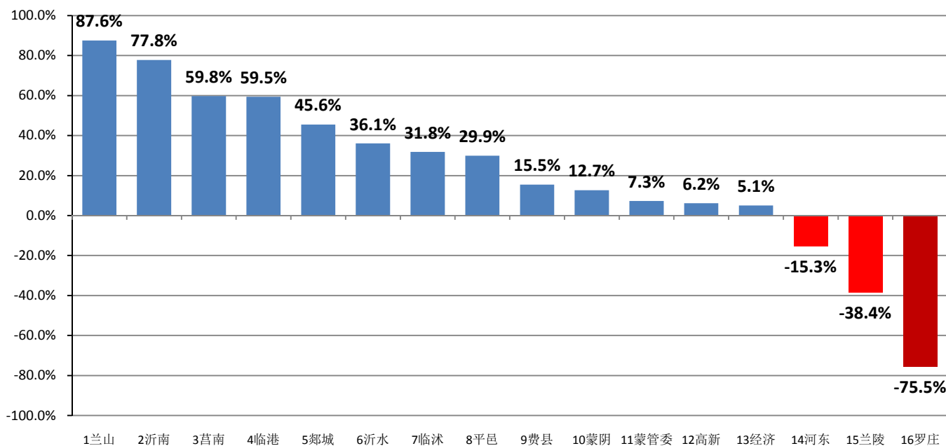
图 4 各县区氨氮同比改善幅度
