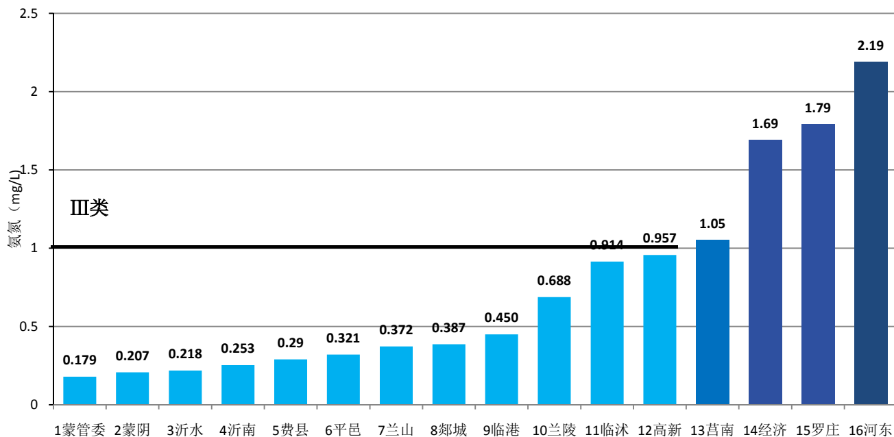
图 3 各县区氨氮浓度排名
