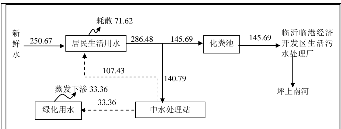
图1 项目灌溉期给排水平衡图 (t/d)
