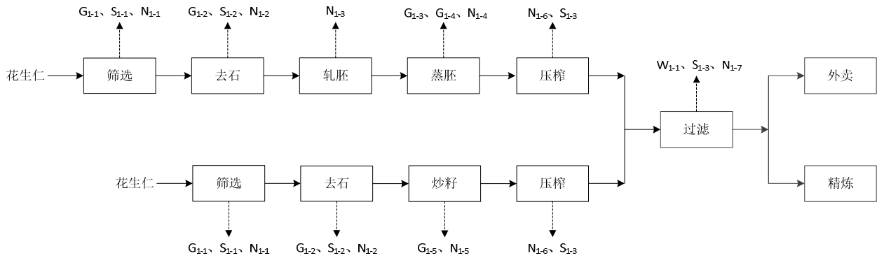
图 7 本项目毛油生产工艺及产污环节图
