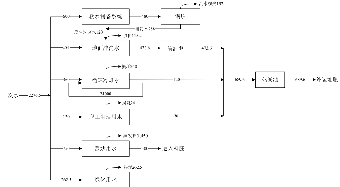
图 3 本项目水平衡图 单位：m 3 /a
