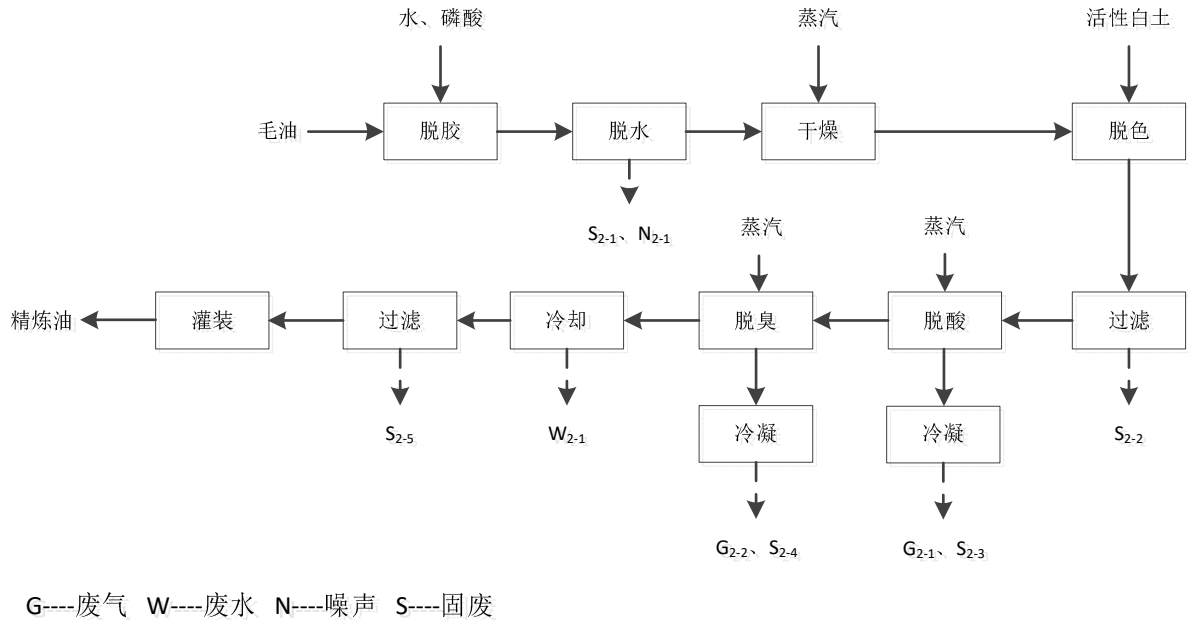
图 8 本项目花生油精炼生产工艺及产排污环节图
